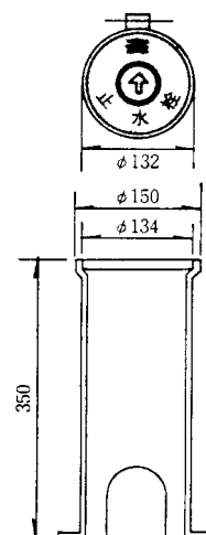
(ケ) 止水栓ボックス(II 型)
