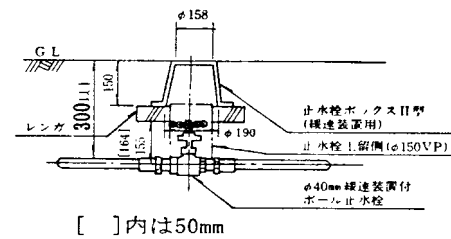
(エ) 止水栓ボックス(Ⅱ型)
