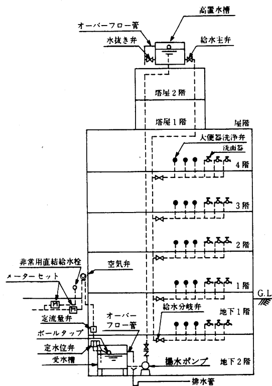
高置水槽方式の一例
