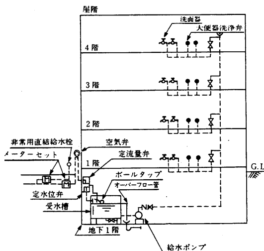
ポンプ直送方式の一例
