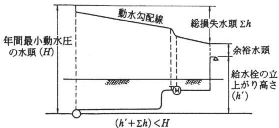
動水勾配線図
