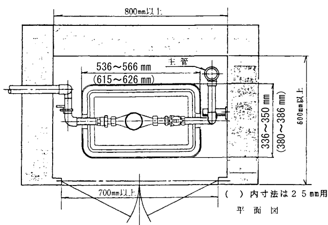
ク パイプシャフト用メーターボックス（口径13mm、20mm、25mm用）設置図
