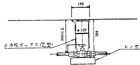
(イ) 止水栓ボックス(乙)
