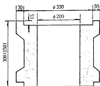
コンクリート製土留側・土留板 (旧版)
