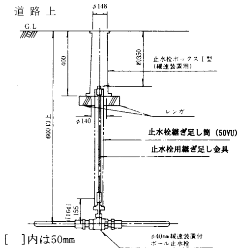
(ウ) 止水栓ボックス(Ⅰ型)
