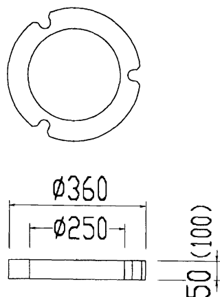
調整リング φ250
