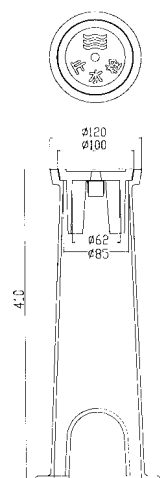
(キ) 止水栓ボックス(樹脂製) [ ] は φ40・50mm 用
