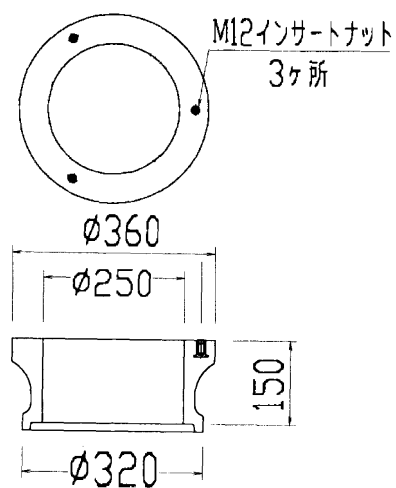
上部土留側 φ250
