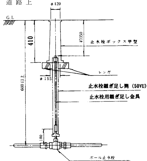
(7) 止水栓ボックス(甲)
