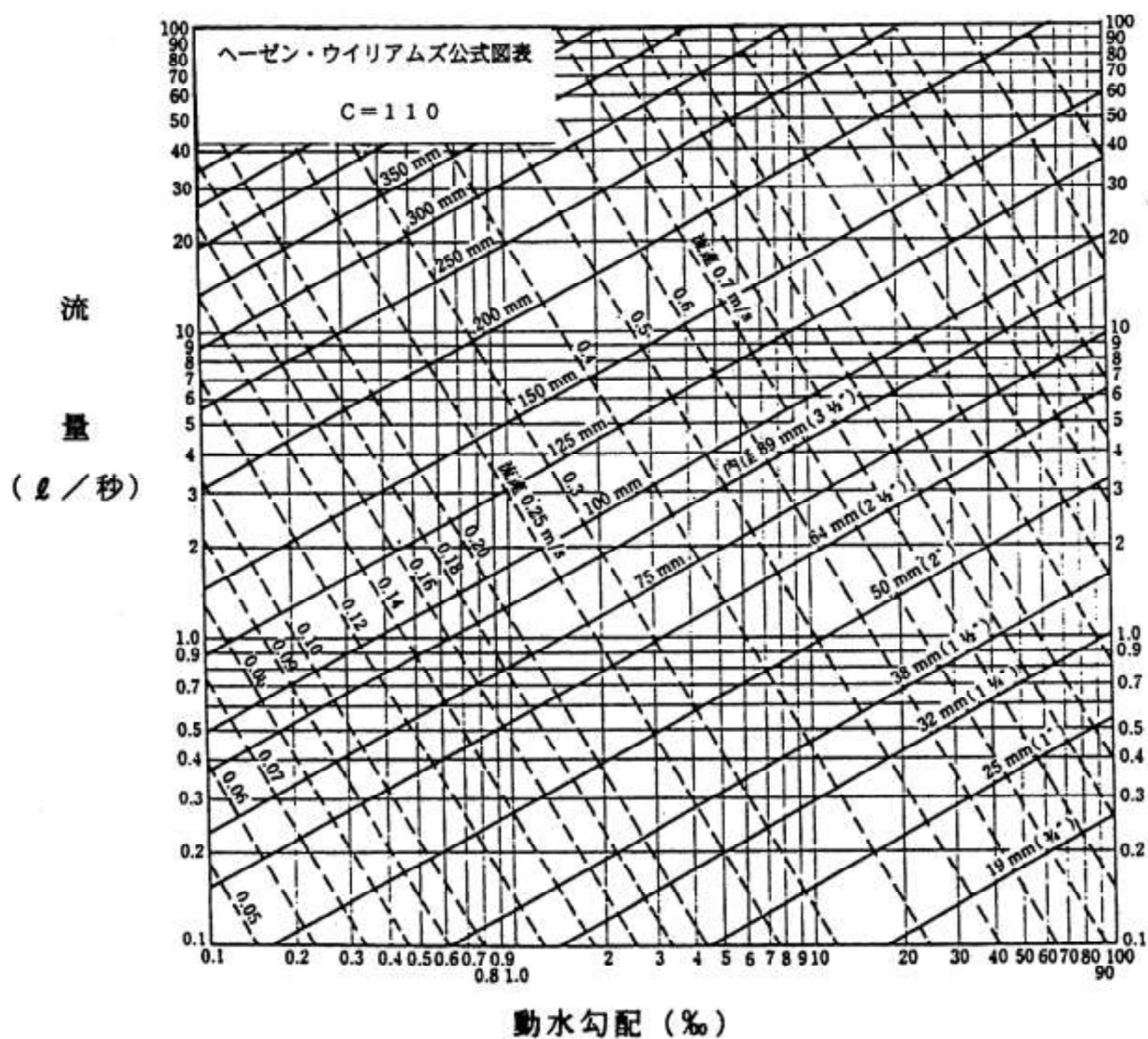
流量曲線図
