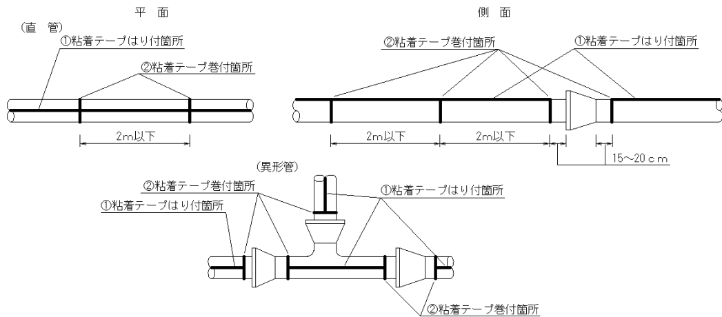
図 3-12 管明示粘着テープ施工方法（口径 75mm～450mm）
