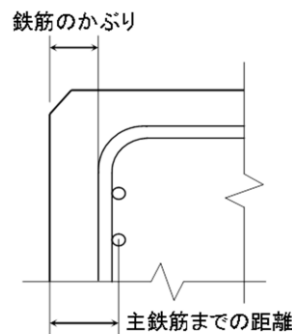
図5-1 鉄筋のかぶり
