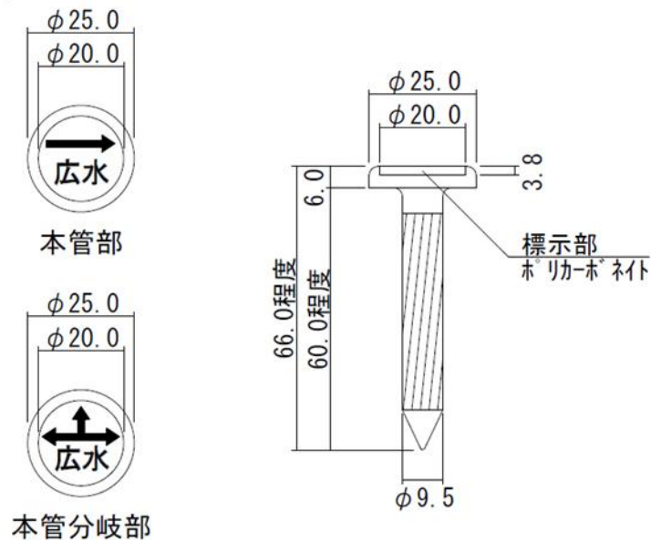
図 3-17 地下埋設物標示鋏（単位:mm）
