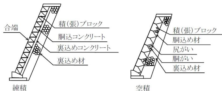
図3-5 コンクリートブロック工
