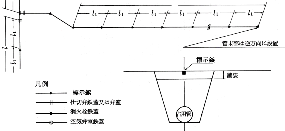
図 3-18 地下埋設物標示板設置位置参考図
