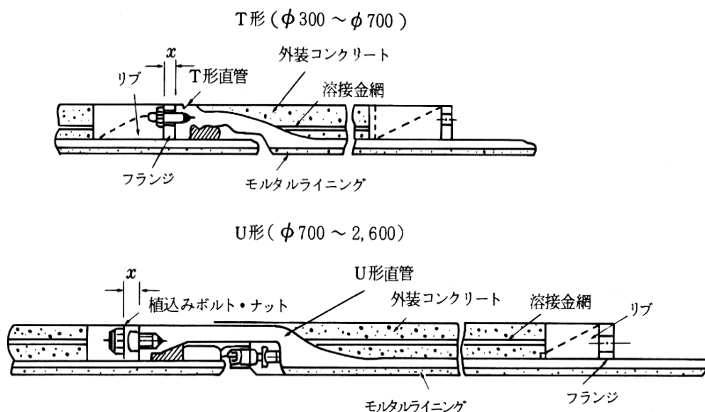
図 3-21 推進工法用ダクトイル管の構造
