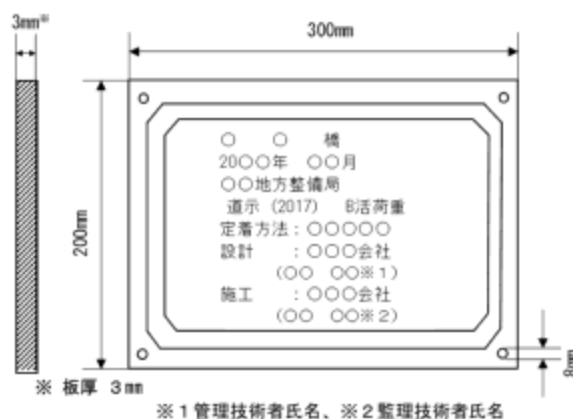
図3-2 銘板の寸法及び記載事項
