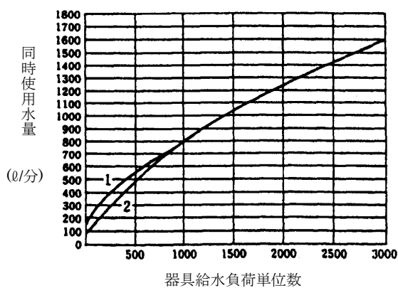
メーター口径選定曲線図 (口径 40 mm 以上)
