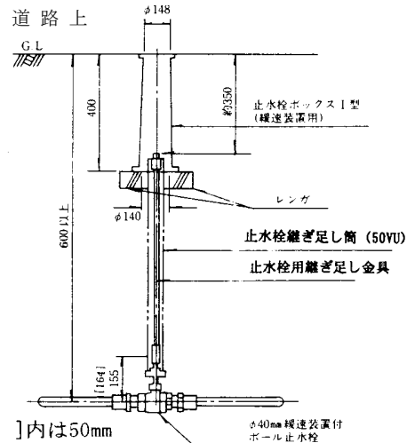
(ウ) 止水栓ボックス(I型)
