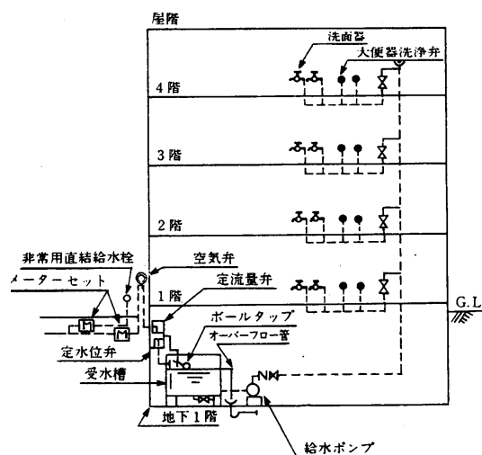
ポンプ直送方式の一例
