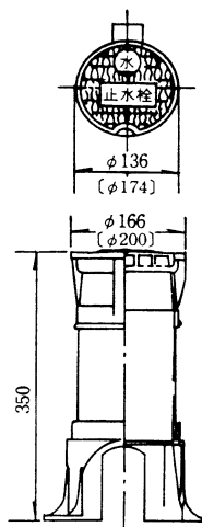
(キ) 止水栓ボックス(樹脂製) [ ] は \phi 40 \cdot 50\text{mm} 用
