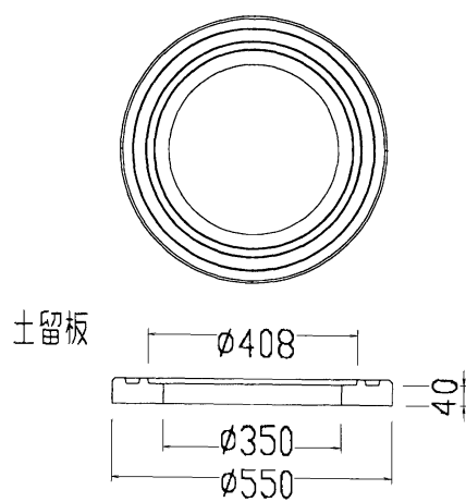
(サ) 仕切弁土留板
