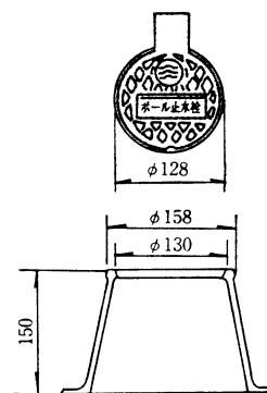
(ケ) 止水栓ボックス(II型)
