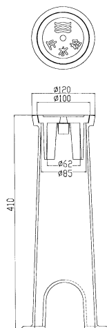
(キ) 止水栓ボックス(樹脂製) [ ] は \phi 40 \cdot 50\text{mm} 用
