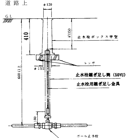
(ア) 止水栓ボックス(甲)
