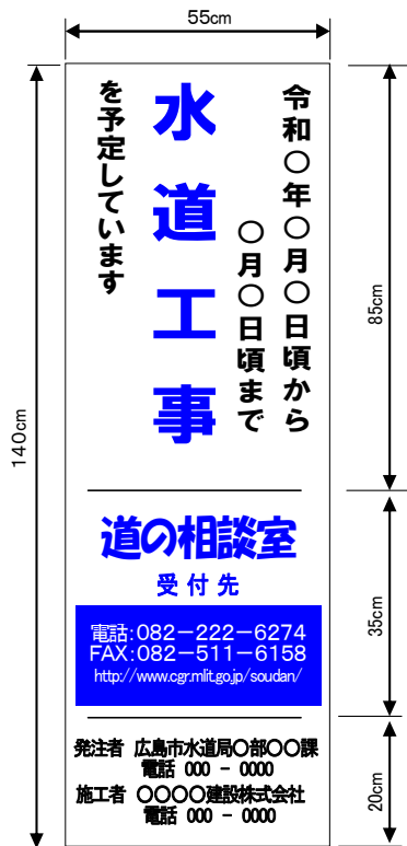
別表様式－ 7 工事情報看板 (水道工事標示例)
