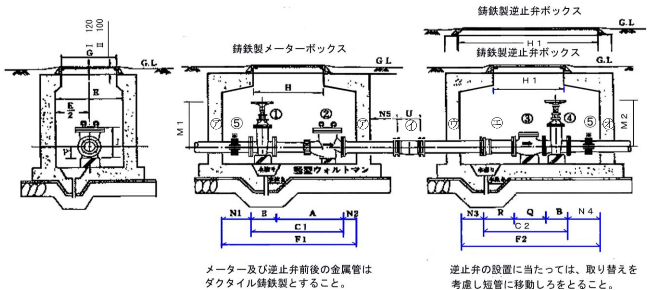
メーターボックスの寸法表
