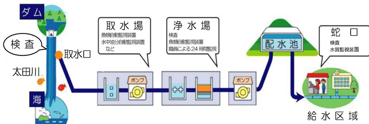
水源から蛇口に至るまでの水質監視体制
