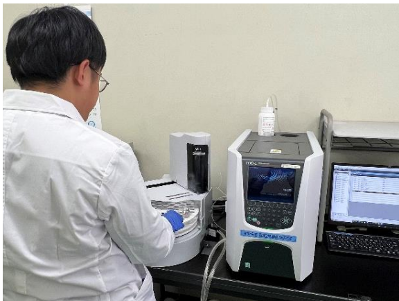
有機物(全有機炭素の量)の検査 (全有機炭素計)
