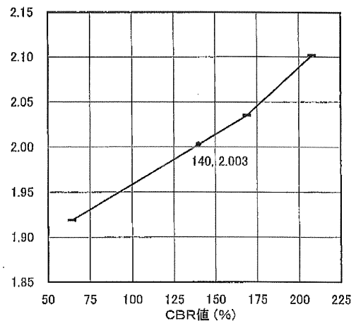
・ CBR—乾燥密度曲線
