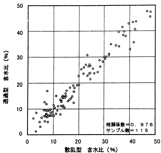
図一11 散乱型と透過型の相関 (含水比・全データ)
