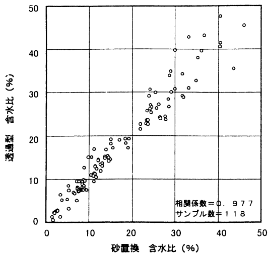
図一七 砂置換と透過型の相関（含水比・全データ）
