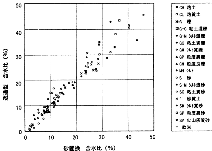
図一八 砂置換と透過型の相関（含水比・土質別データ）
