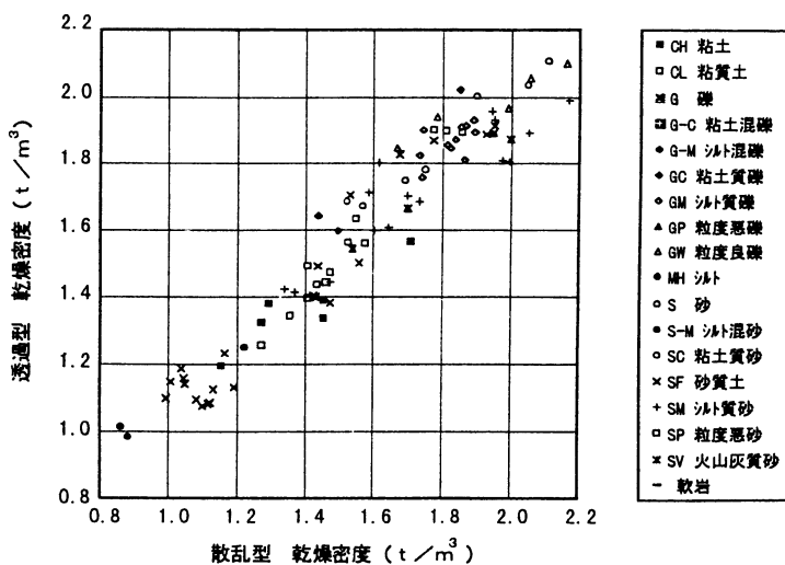
図一〇 散乱型と透過型の相関 (乾燥密度・土質別データ)
