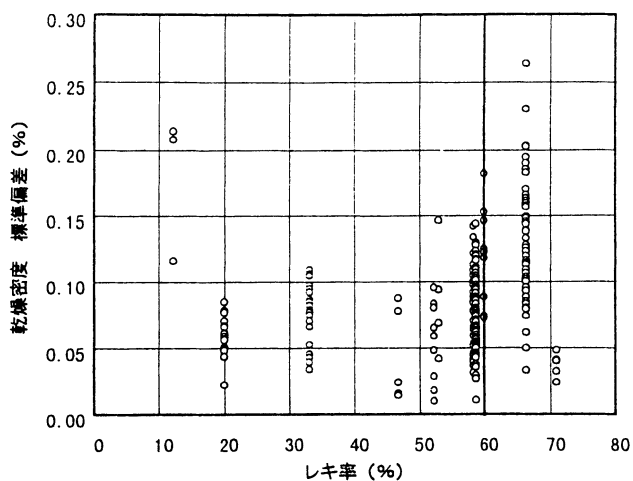
図一13 レキ率と乾燥密度（標準偏差）の関係〔散乱型〕
