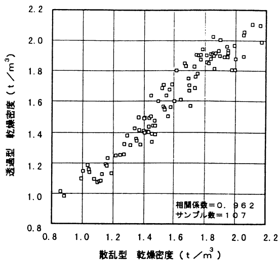
図一 散乱型と透過型の相関 (乾燥密度・全データ)
