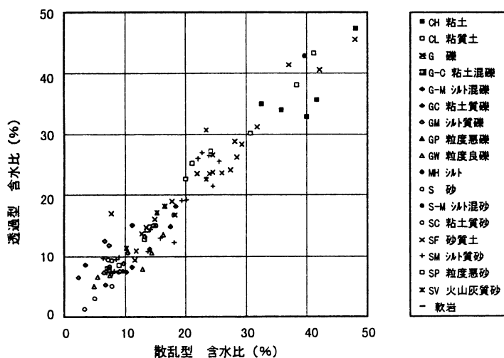
図一12 散乱型と透過型の相関 (含水比・土質別データ)
